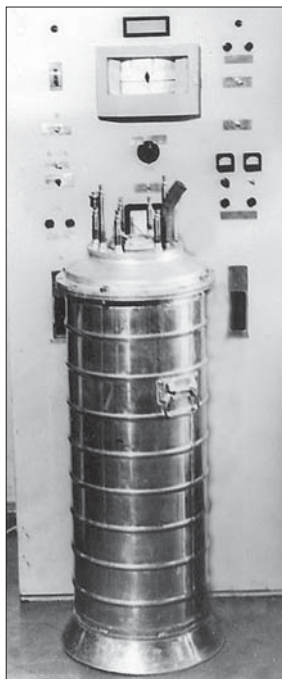
Фото 5. Гелієвий кріостат з надпровідним магнітним екраном з діаметром вхідного отвору 150 мм для метрологічних випробувань надпровідних квантових магніметрів
